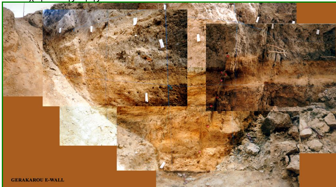
Εικόνα 2-22. Συνθετική εικόνα του ανατολικού τοιχώματος της παλαιοσεισμολογικής τομής GER-4 (παράταξη τομής B-N) στην οποία διακρίνεται η ρηξιγενής ζώνη.
