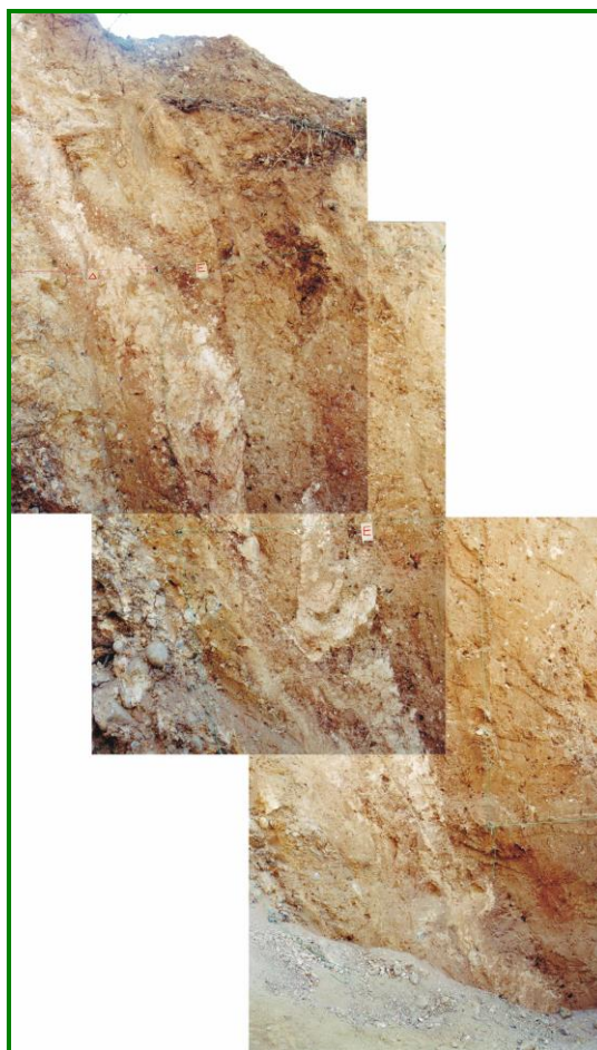
Εικόνα 3-18. Σύνθετη απεικόνιση λεπτομέρειας της ρηξιγενούς ζώνης στην παλαιοσεισμολογική τομή ΚΑΡ-1.
