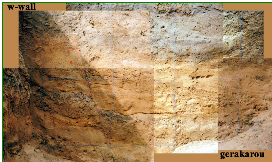
Εικόνα 2-23. Συνθετική εικόνα τμήματος του δυτικού τοιχώματος της παλαιοσεισμολογικής τομής GER-4 (παράταξη τομής N-B). Διακρίνεται η ρηξιγενής ζώνη, η οποία ταυτίζεται με τη σεισμική διάρρηξη του 1978.
