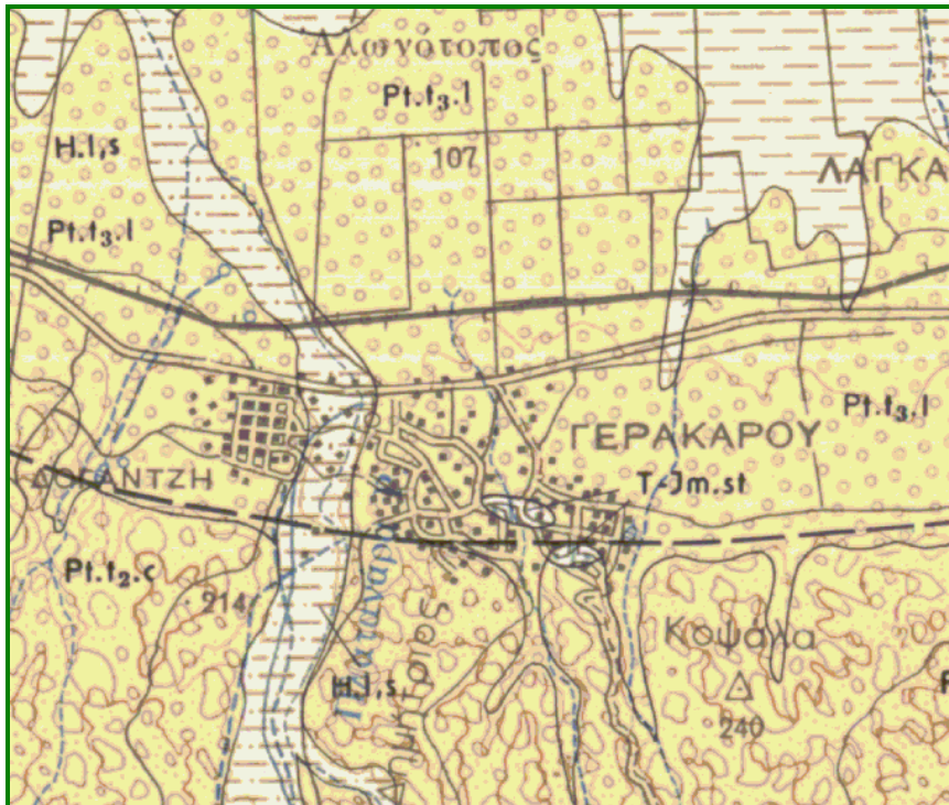
Εικόνα 2-14. Λεπτομέρεια του γεωλογικού χάρτη του Ι.Γ.Μ.Ε. κλίμακας 1:50.000 της περιοχής της Γερακαρούς. Η.Ι,ς: αποθέσεις στις κοίτες χειμάρρων – αμμούχες άργιλοι, άμμοι και ψηφίδες (Ολόκαινο), Pt.t3.l: κατώτερο σύστημα αναβαθμίδων – χαλίκια και άμμοι (Πλειστόκαινο), Pt.t2.c: μεσαίο σύστημα αναβαθμίδων ή «Σχηματισμός Γερακαρούς»– άμμοι και χαλίκια (Αν. Πλειόκαινο – Βιλλαφράγκιο), T-Jm.st: χαλαζίτες του «φλύσχη της Σβούλας» (Τριαδικό – Μέσο Ιουρασικό).
