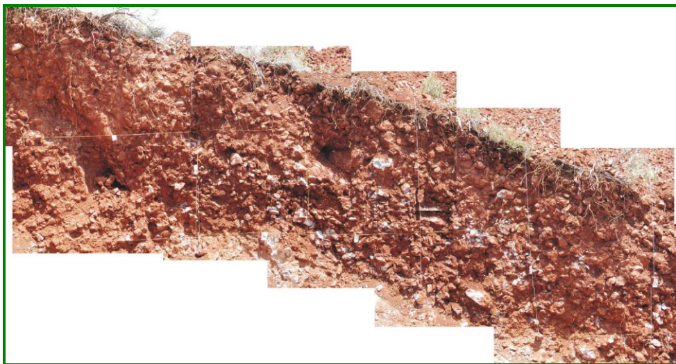
Εικόνα 3-22. Σύνθετη απεικόνιση λεπτομέρειας του ανατολικού τοιχώματος της παλαιοσεισμολογικής τομής ΚΑΡ-3.
