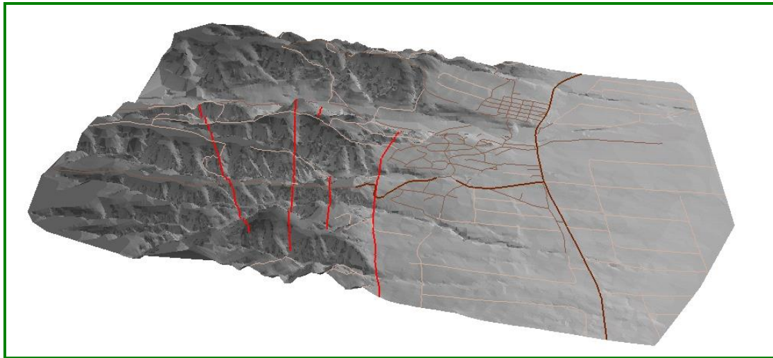
Εικόνα 2-7. Τρισδιάστατη υπερυψωμένη απεικόνιση της μορφολογίας στην περιοχή της Γερακαρούς. Διακρίνονται τα χαρτογραφημένα κανονικά ρήγματα (κόκκινες γραμμές) και το οδικό δίκτυο. Όψη προς τα Δ.
