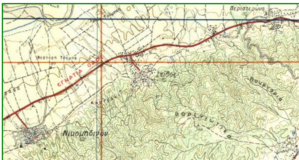
Εικόνα 2-27. Τοπογραφία στην ευρύτερη περιοχή του Στίβου. Διακρίνεται η διαφορά στη μορφολογία
